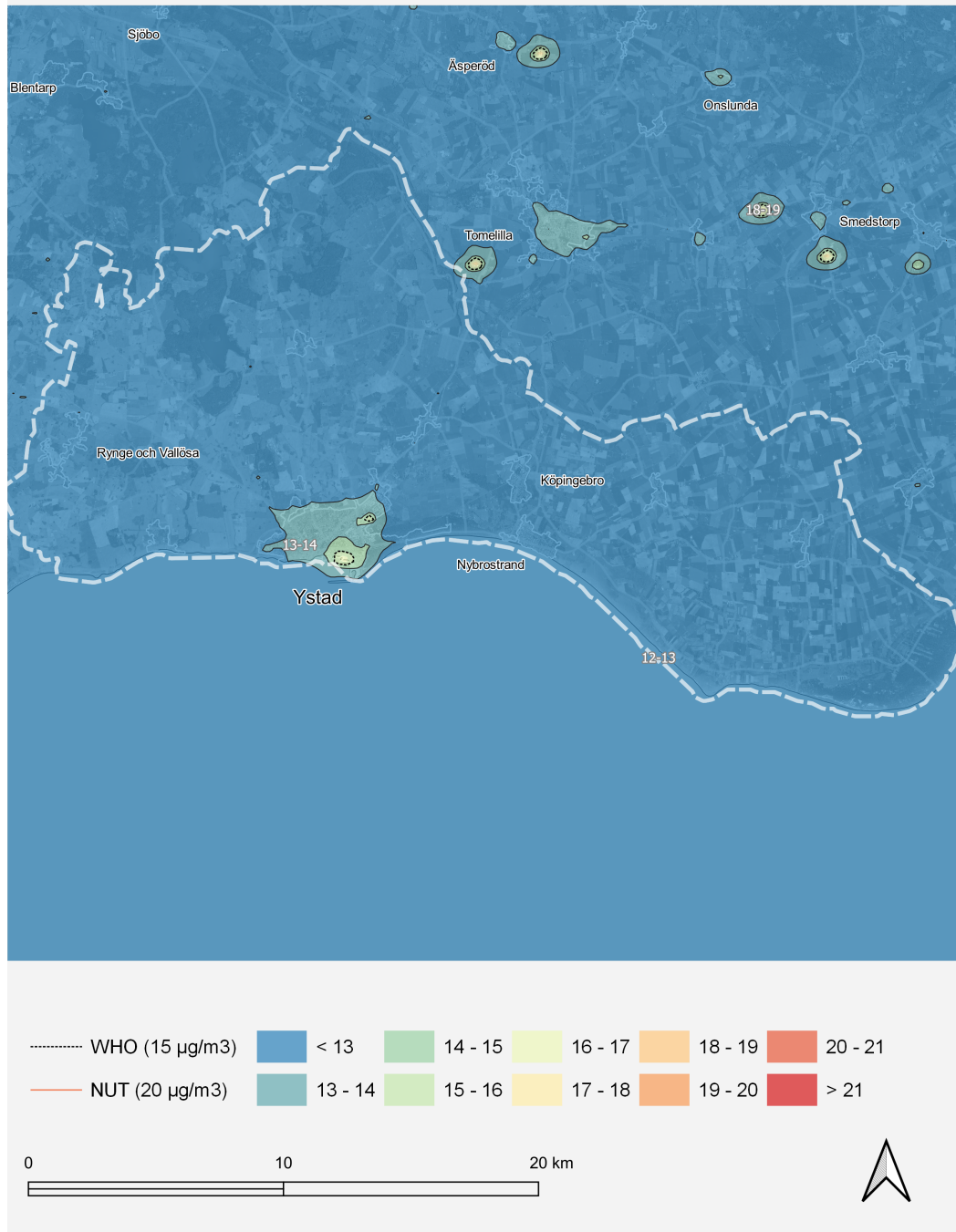
Figur 9. Karta som visar årsmedelvärdet av PM10 för år 2021 i Ystad.
