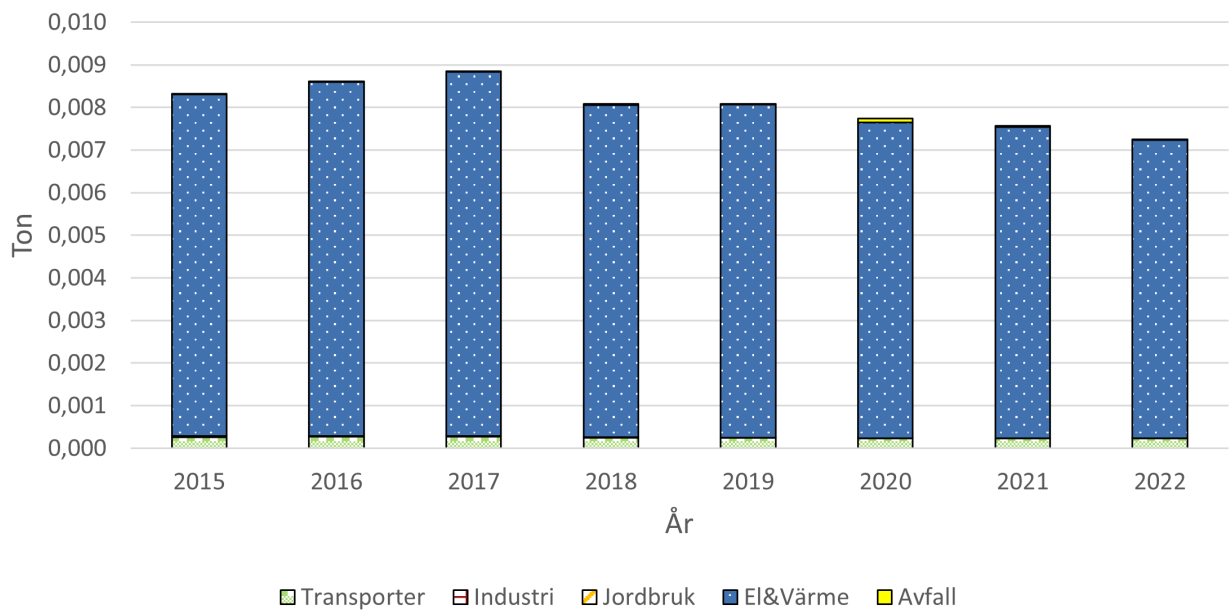
Figur 19. Visar utsläppskällorna av PAH för Ystad, vilket inkluderar bens(a)pyren. beräknat värde från SMHI.
