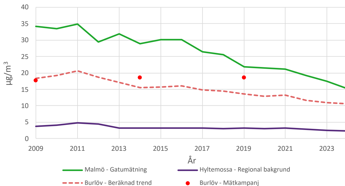
Figur 2. Visar mätningar av \text{NO}_2 samt en extrapolerad trend på förändringen mellan år 2009 – 2024. Jämfört med Malmö och bakgrundsmätningar Hyltemossa.
