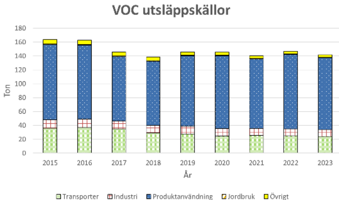
Figur 27. Visar utsläppskällorna av VOC, beräknat värde från SMHI.
