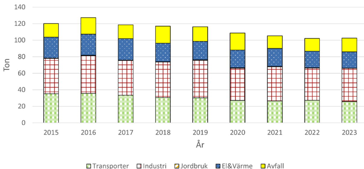
Figur 19. Visar utsläppskällorna av PM2.5, beräknat värde från SMHI.
