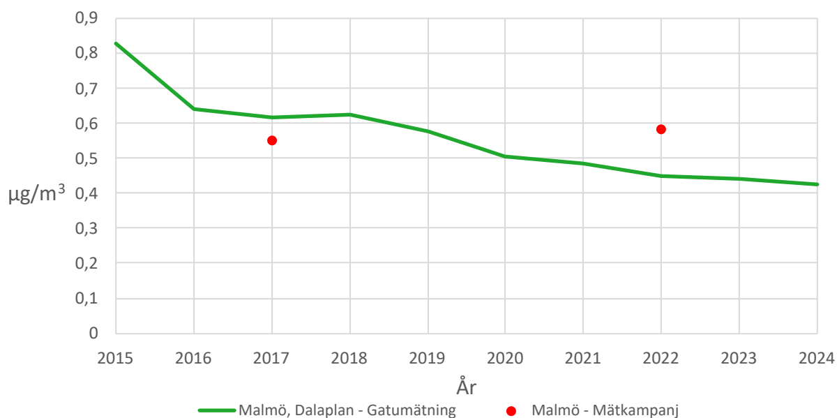
Figur 26. Visar beräknade halter av bensen för år 2024 baserad på mätkampanjer år 2017 och 2022.
