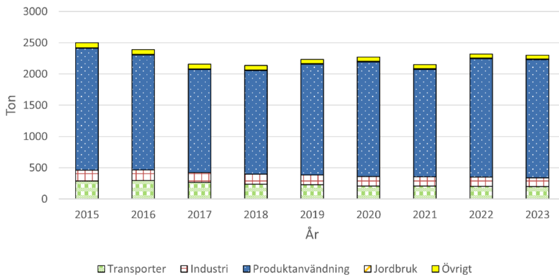
Figur 27. Visar utsläppskällorna av VOC, beräknat värde från SMHI.
