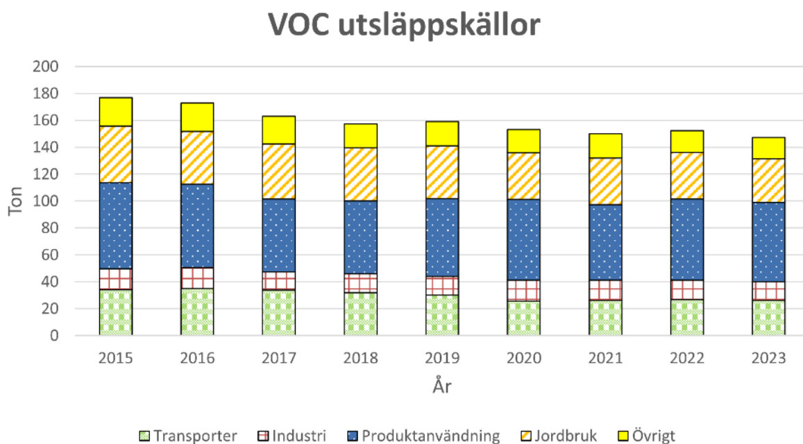
Figur 27. Visar utsläppskällorna av VOC, beräknat värde från SMHI.
