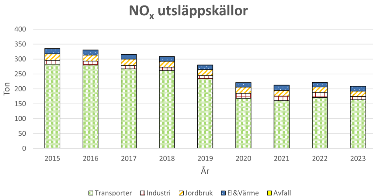
Figur 7. Visar utsläppskällorna av NO x , beräknat värde från SMHI.
