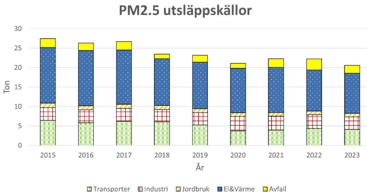
Figur 19. Visar utsläppskällorna av PM2.5, beräknat värde från SMHI.
