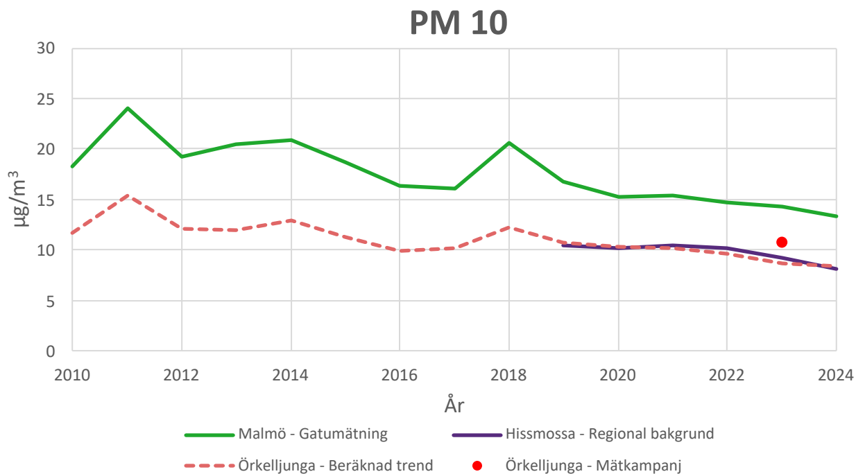
Figur 12. Visar mätningar av PM10 samt en extrapolerad trend på förändringen mellan år 2012 – 2024. Jämförs med gatumätning i Malmö samt regional bakgrund i Hissmossa.
