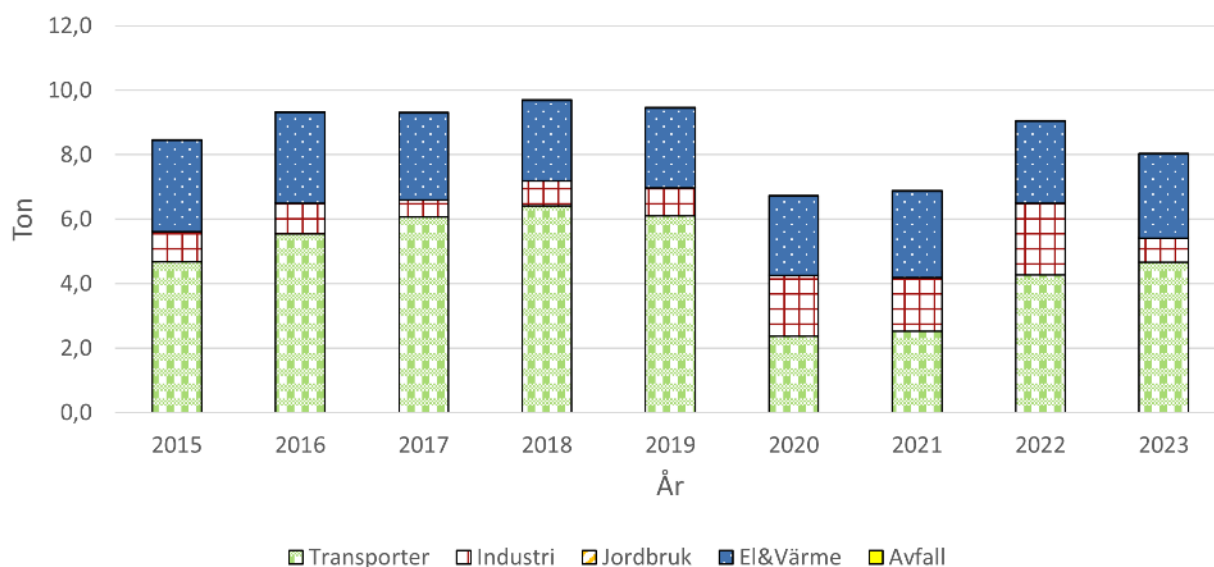
Figur 15. Visar utsläppskällorna av PM 10 , beräknat värde från SMHI.
