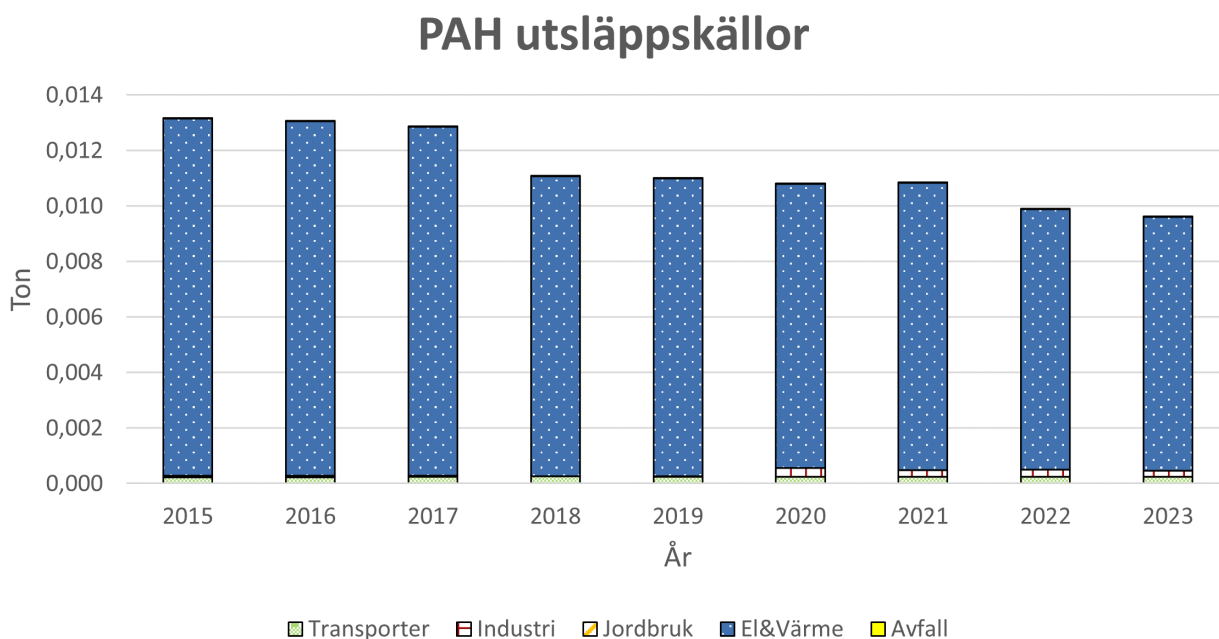
Figur 25. Visar utsläppskällorna av PAH, vilket inkluderar bens(a)pyren. beräknat värde från SMHI.
