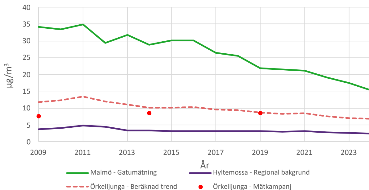
Figur 2. Visar mätningar av NO 2 samt en extrapolerad trend på förändringen mellan år 2009 – 2024. Jämfört med Malmö och bakgrundsmätningar Hyltemossa.
