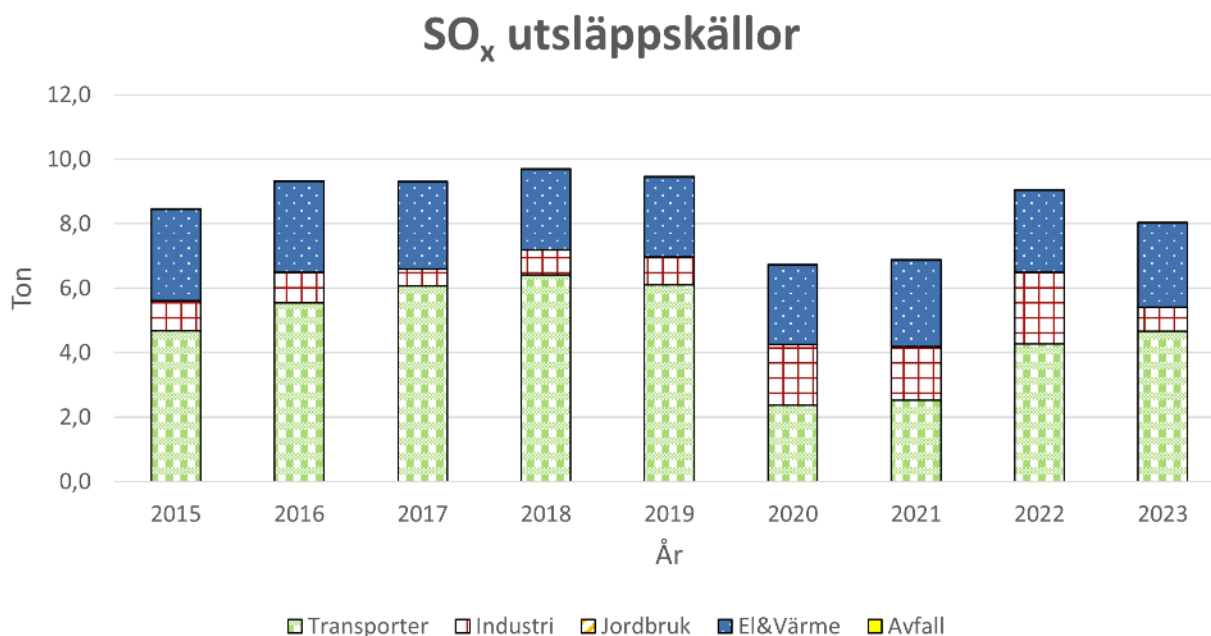
Figur 11. Visar utsläppskällorna av SO x , beräknat värde från SMHI.
