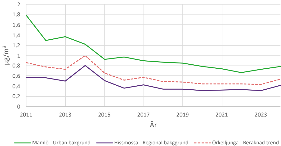
Figur 8. Visar mätningar av SO 2 samt en extrapolerad trend på förändringen mellan år 2011 – 2024. Jämförs med mätningar i urban bakgrund i Malmö samt regional bakgrund i Hissmossa.
