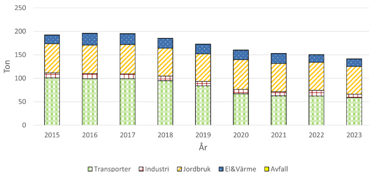
Figur 7. Visar utsläppskällorna av NO x , beräknat värde från SMHI.
