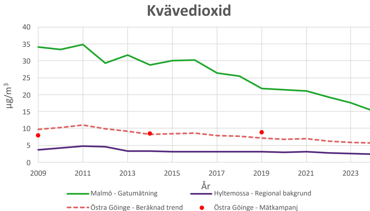
Figur 2. Visar mätningar av \text{NO}_2 samt en extrapolerad trend på förändringen mellan år 2009 – 2024. Jämfört med Malmö och bakgrundsmätningar Hyltemossa.
