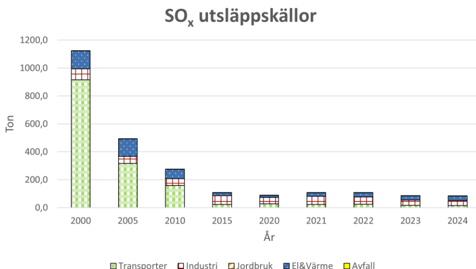
Figur 9. Visar utsläppskällorna av SO x , beräknat värde från SMHI.
