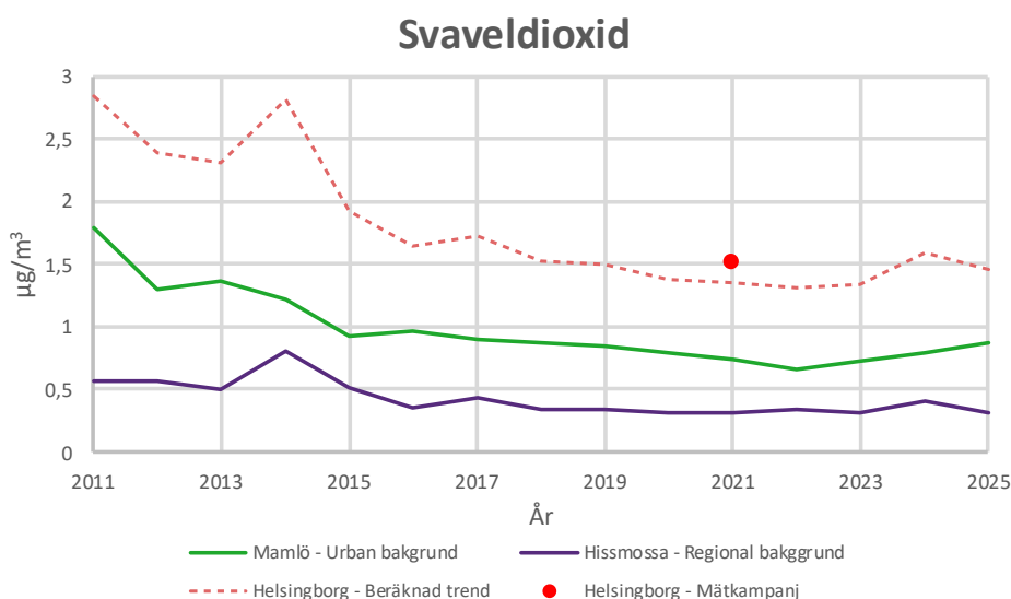
Figur 6. Visar trenden av SO 2 mellan 2011 – 2025. Jämförs med mätningar i urban bakgrund i Malmö samt regional bakgrund i Hissmossa.
