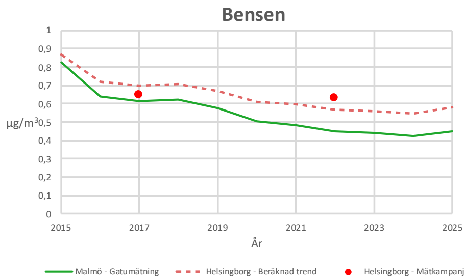
Figur 24. Visar beräknade halter av bensen för år 2024 baserad på mätkampanjer år 2017 och 2022.
