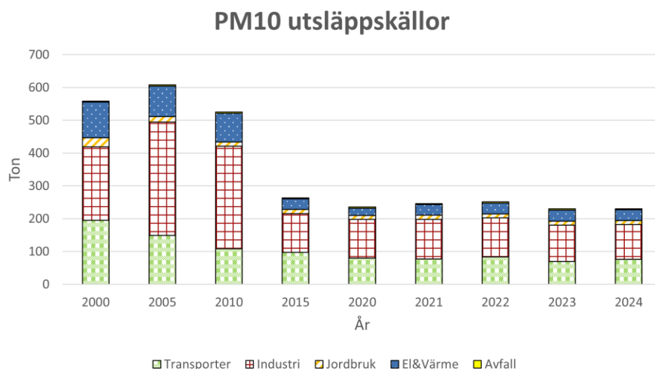
Figur 13. Visar utsläppskällorna av PM10, beräknat värde från SMHI.
