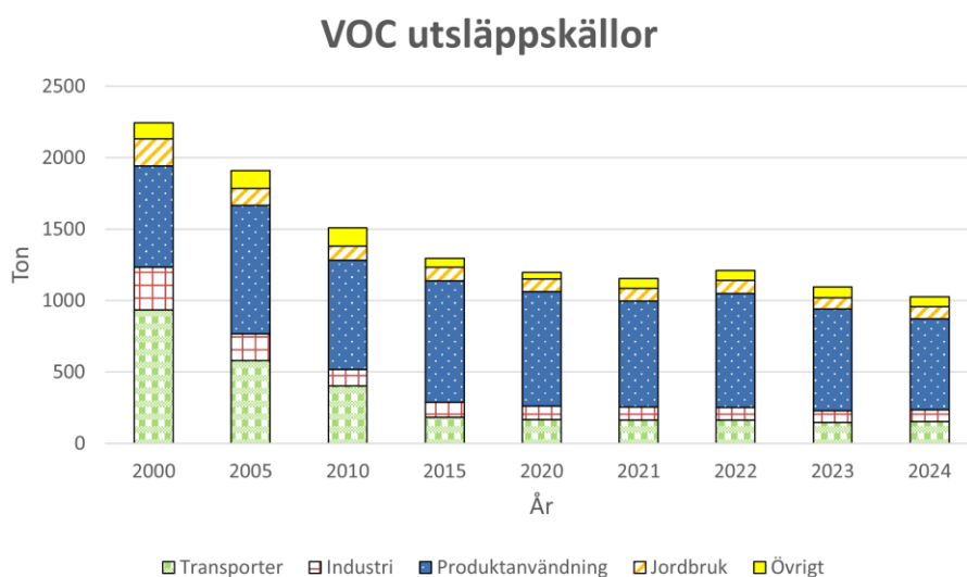
Figur 25. Visar utsläppskällorna av VOC, beräknat värde från SMHI.
