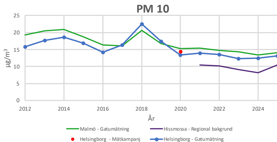
Figur 10. Visar trenden av PM10 mellan 2010 – 2025. Jämförs med mätningar i gaturum i Malmö samt regional bakgrund i Hissmossa.
