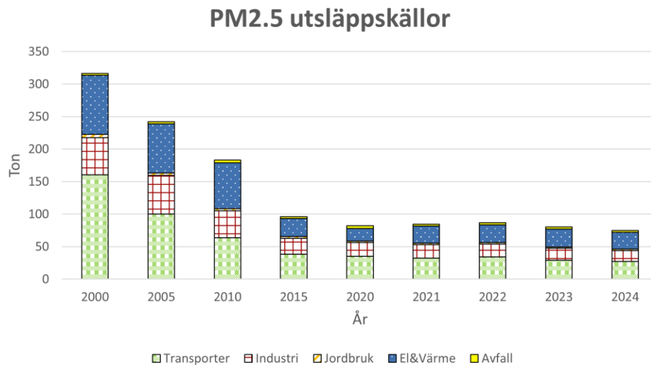
Figur 17. Visar utsläppskällorna av PM2.5, beräknat värde från SMHI.
