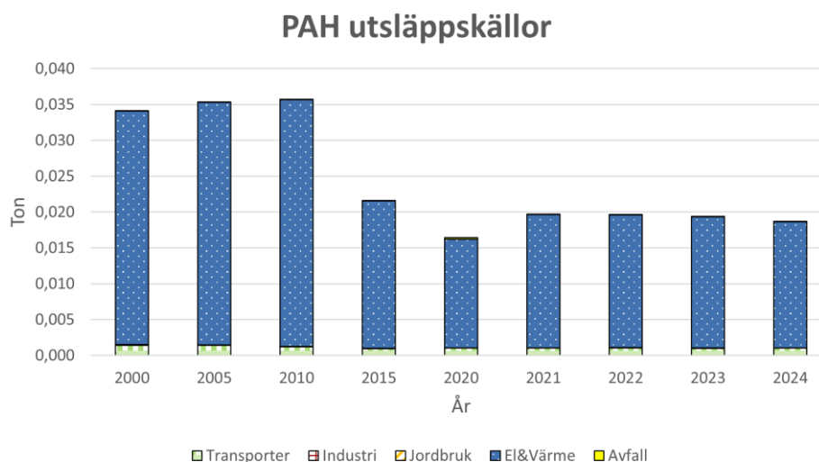
Figur 23. Visar utsläppskällorna av PAH, beräknat värde från SMHI.
