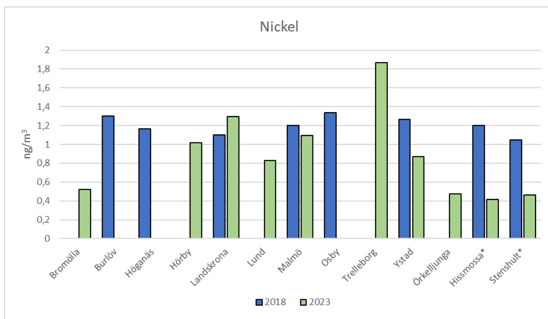
Figur 21. Medelkoncentrationen av nickel i tio kommuner och två bakgrundstationer (*) under mätkampanjer år 2018 & 2023.
