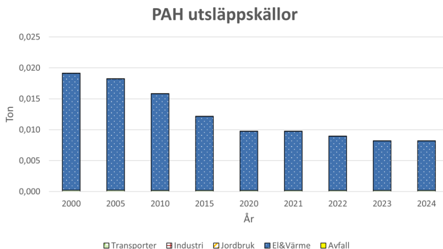
Figur 20. Visar utsläppskällorna av PAH, beräknat värde från SMHI.
