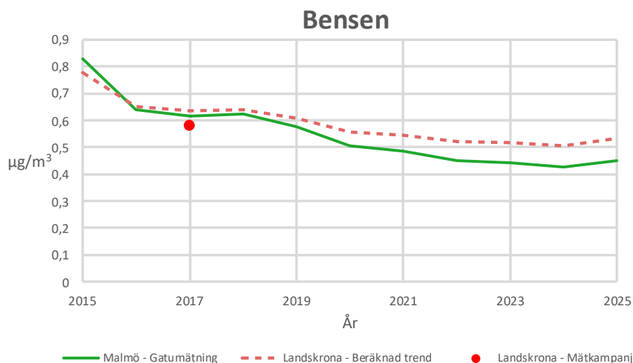
Figur 23. Visar beräknade halter av bensen för år 2024 baserad på mätkampanjer år 2017 och 2022.
