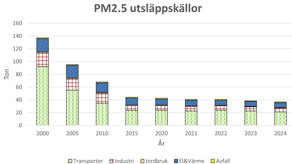
Figur 16. Visar utsläppskällorna av PM2.5, beräknat värde från SMHI.
