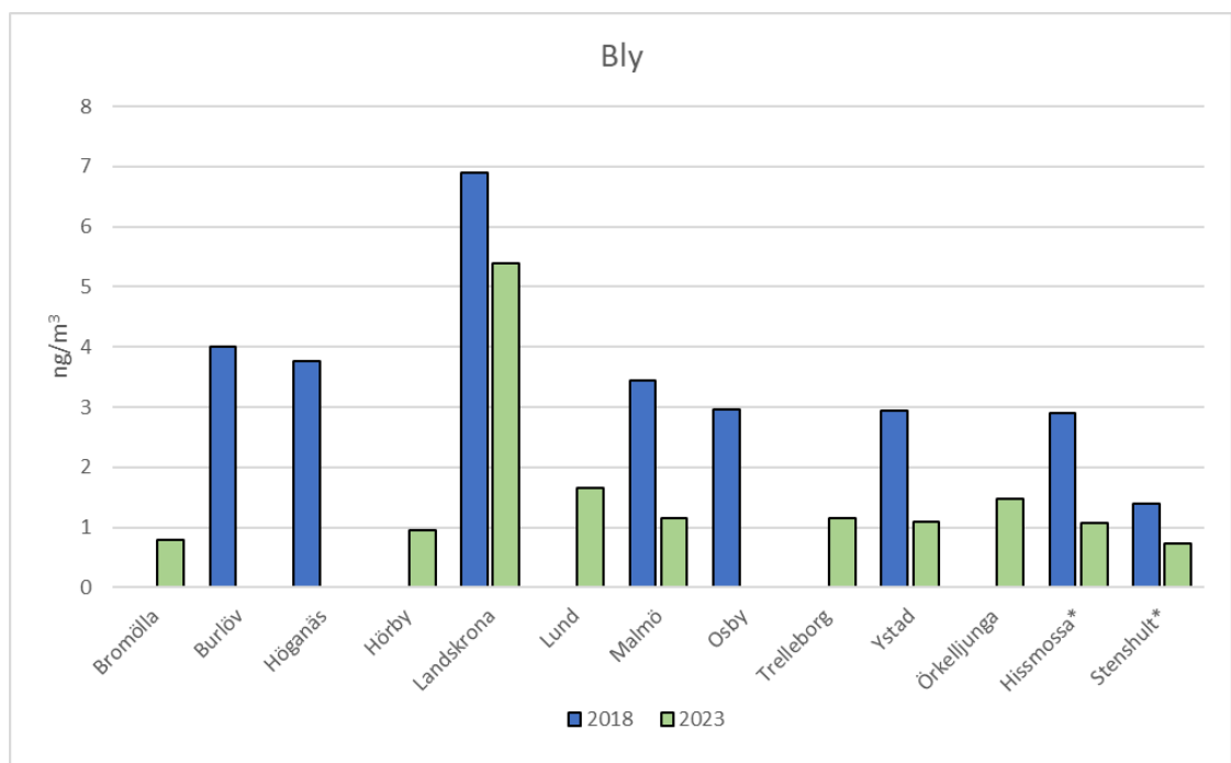
Figur 18. Medelkoncentrationen av bly i tio kommuner och två bakgrundstationer (*) under mätkampanjer år 2018 & 2023.
