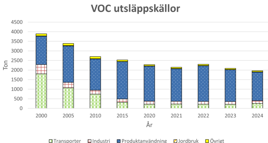
Figur 25. Visar utsläppskällorna av VOC, beräknat värde från SMHI.
