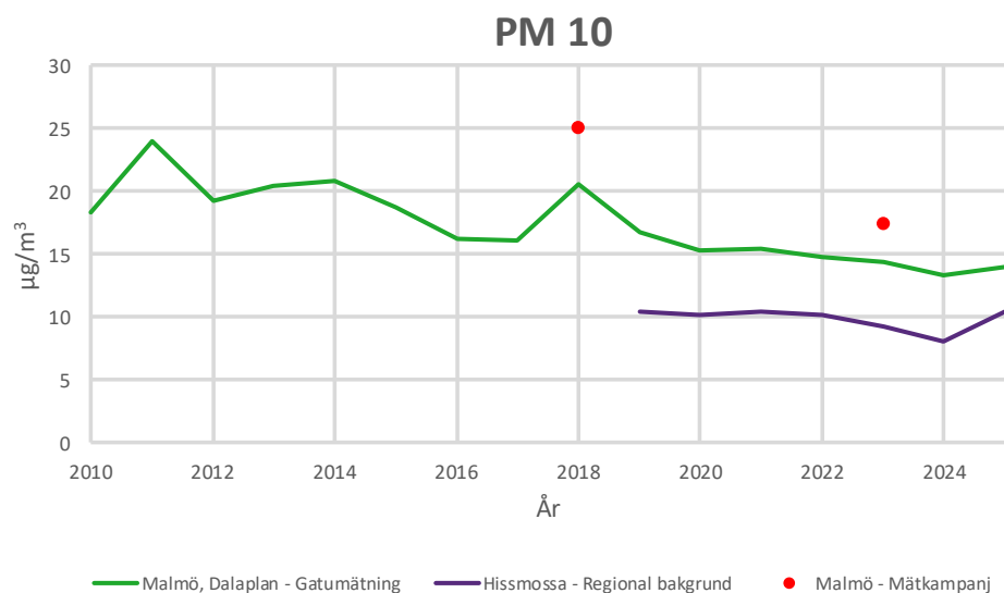
Figur 10. Visar trenden av PM10 mellan 2010 – 2025. Jämförs med mätningar i gaturum i Malmö samt regional bakgrund i Hissmossa.
