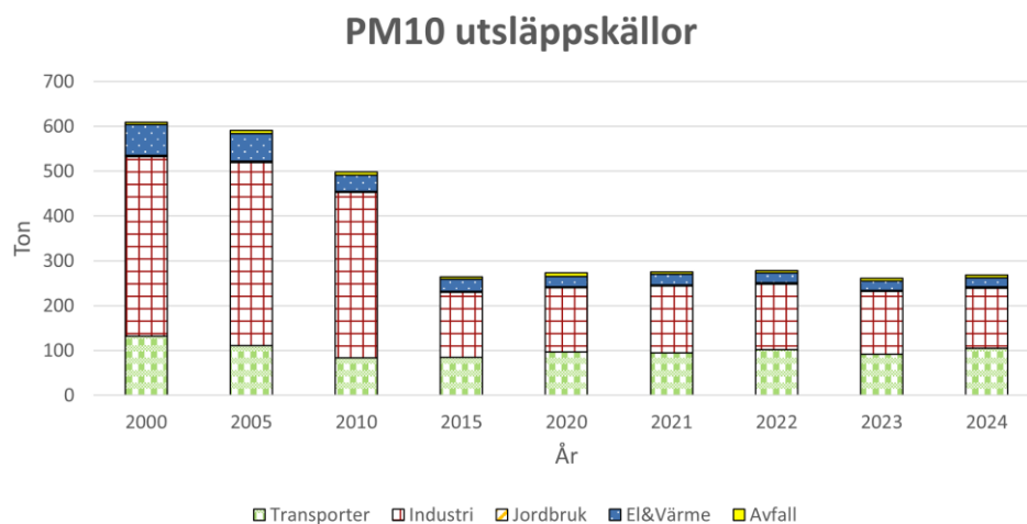
Figur 13. Visar utsläppskällorna av PM10, beräknat värde från SMHI.
