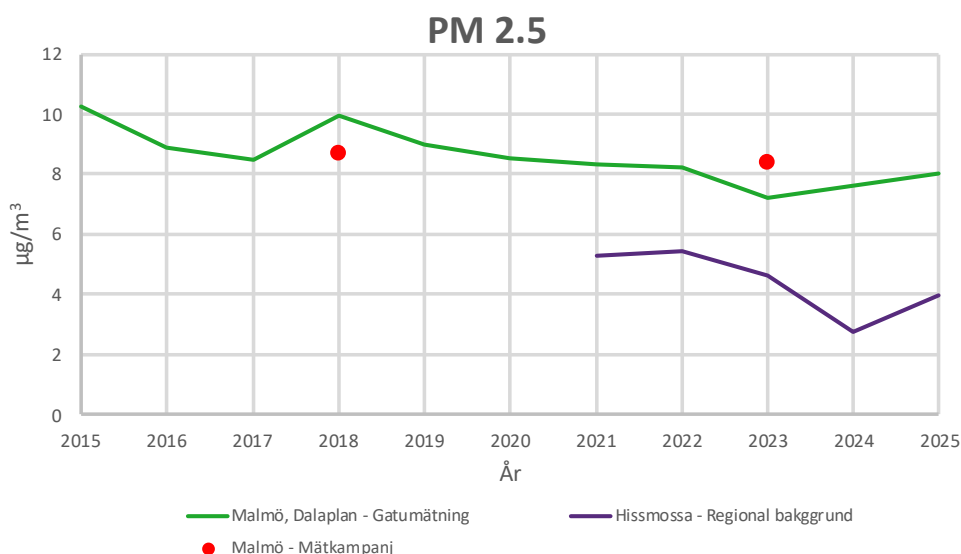
Figur 14. Visar trenden av PM2.5 mellan 2010 – 2025. Jämförs med mätningar i gaturum i Malmö samt regional bakgrund i Hissmossa.
