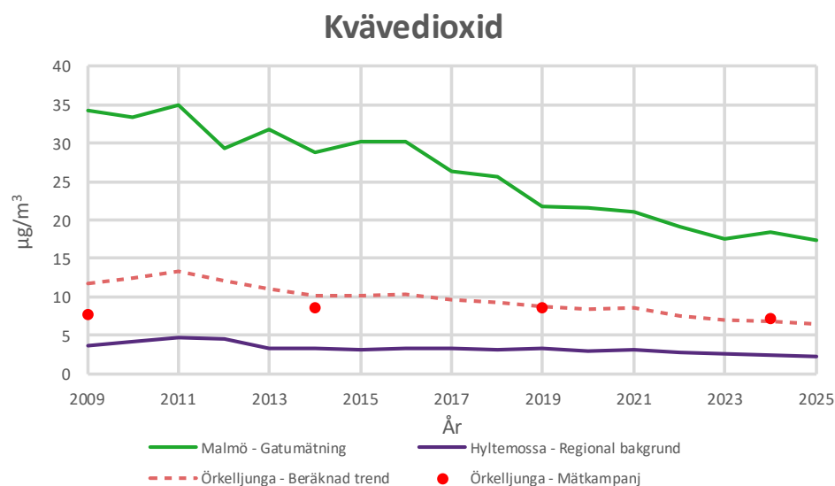
Figur 2. Visar mätningarna av NO 2 samt en extrapolerad trend över förändringen. Trenden jämförs med de kontinuerliga mätningarna i Malmö och Hyltemossa.
