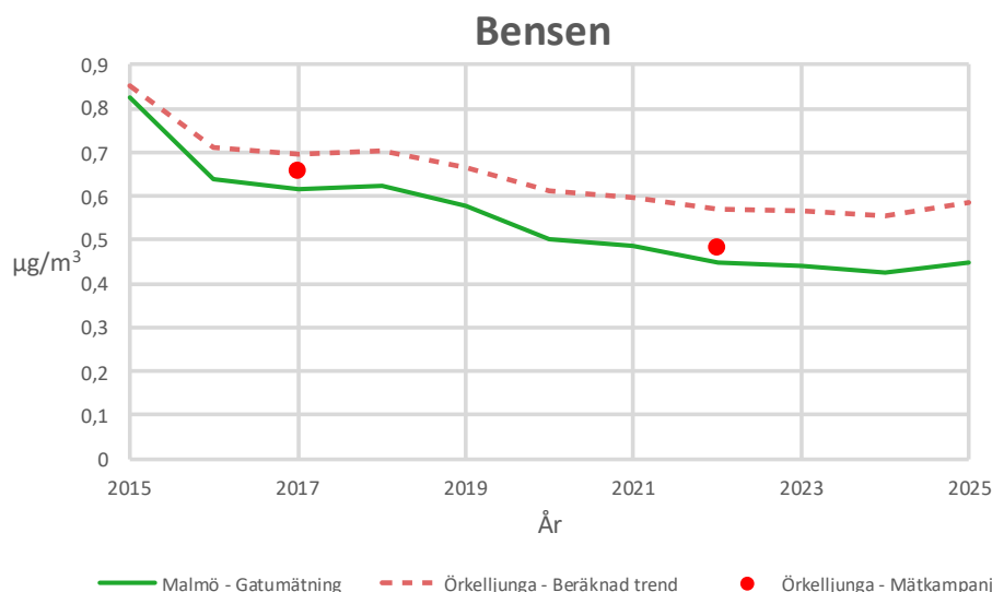
Figur 21. Visar beräknade halter av bensen för år 2024 baserad på mätkampanjer år 2017 och 2022.
