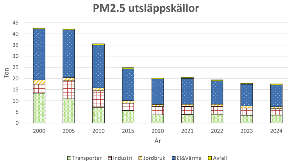
Figur 14. Visar utsläppskällorna av PM2.5, beräknat värde från SMHI.
