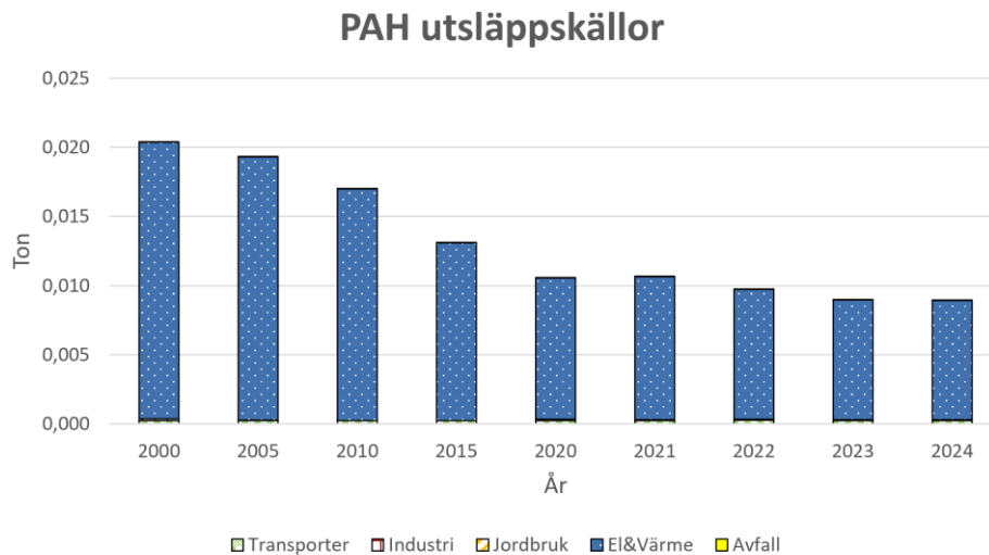
Figur 20. Visar utsläppskällorna av PAH, beräknat värde från SMHI.
