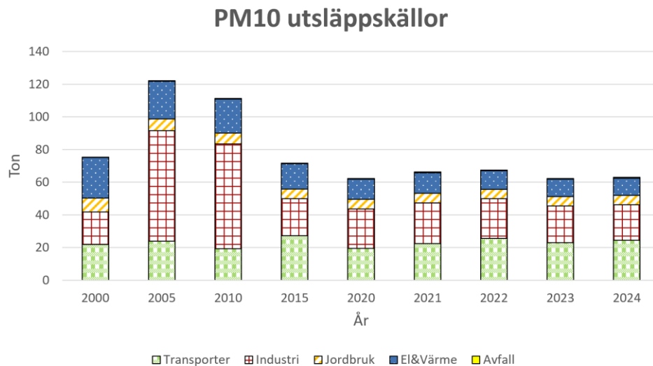
Figur 11. Visar utsläppskällorna av PM10, beräknat värde från SMHI.
