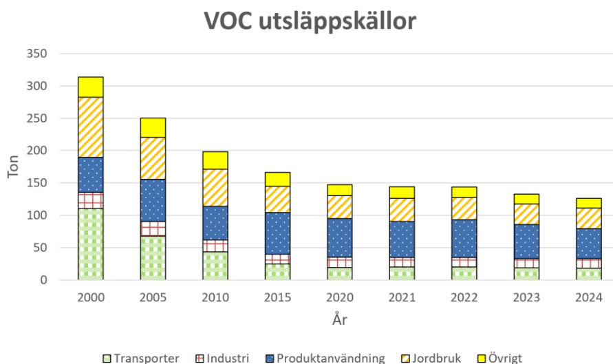
Figur 22. Visar utsläppskällorna av VOC, beräknat värde från SMHI.
