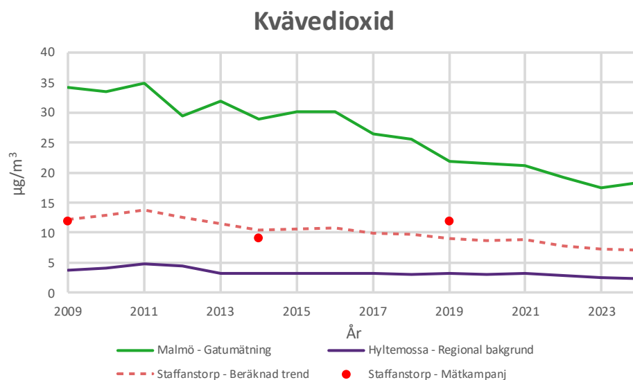
Figur 2. Visar mätningarna av NO 2 samt en extrapolerad trend över förändringen. Trenden jämförs med de kontinuerliga mätningarna i Malmö och Hyltemossa.
