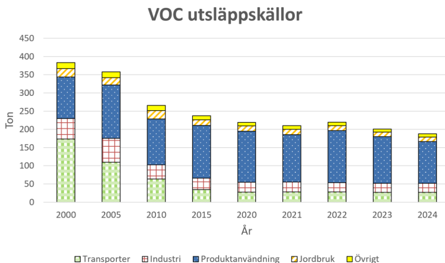
Figur 22. Visar utsläppskällorna av VOC, beräknat värde från SMHI.
