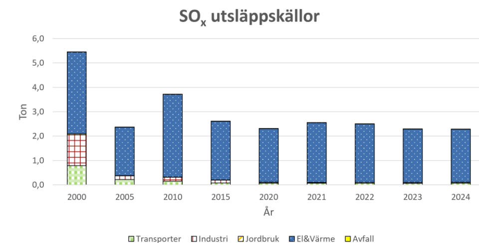
Figur 8. Visar utsläppskällorna av SO x , beräknat värde från SMHI.
